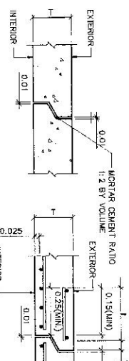
รายละเอียดการต่อกล่องพังก่อนแบบในรูปแสดง ขนาด 1:10
